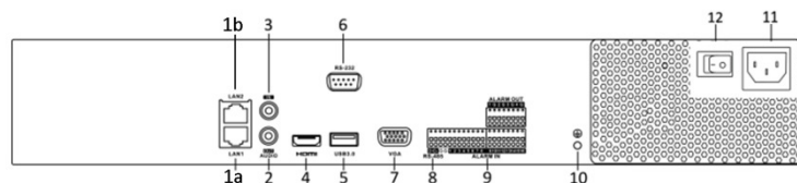
DS-7732NI-I4
